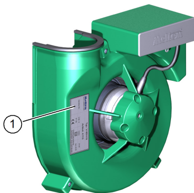
Рис. 1: табличка спецификации на двигателе вентилятора
